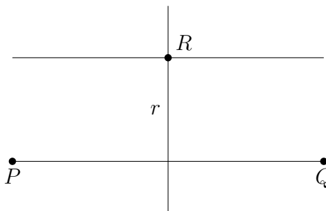
Figura 1.6: Construcción de una recta paralela a otra dada que pase por un punto.
