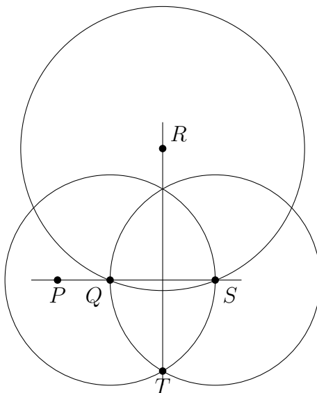
Figura 1.5: Trazar recta perpendicular por R si R no está en la recta PQ .
