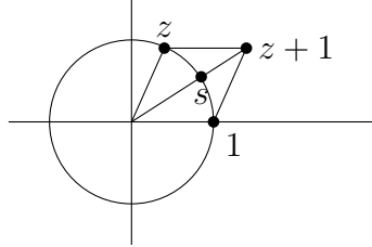
Figura 1.14: Obtención de \sqrt{z} a partir de z .
