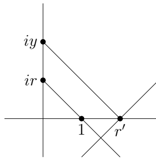
Figura 1.11: Obtención de r \cdot r' a partir de r y r' .
