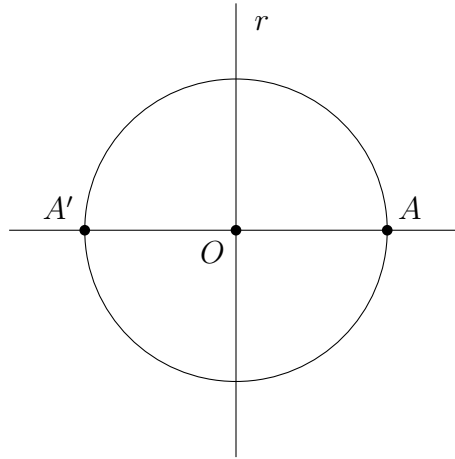
Figura 1.7: Construcción del simétrico de un punto respecto de una recta.
