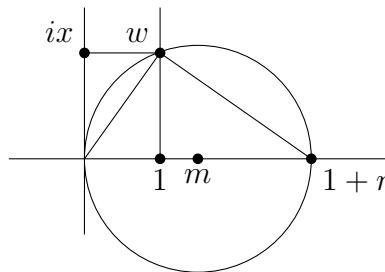
Figura 1.13: Obtención de \sqrt{r} a partir de r .
