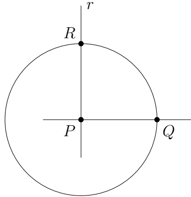
Figura 1.8: Construcción de un sistema de referencia ortonormal.
