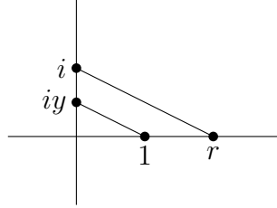
Figura 1.12: Obtención de r^{-1} a partir de r .
