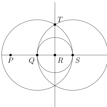
Figura 1.4: Trazar recta perpendicular por R si R está en la recta PQ .
