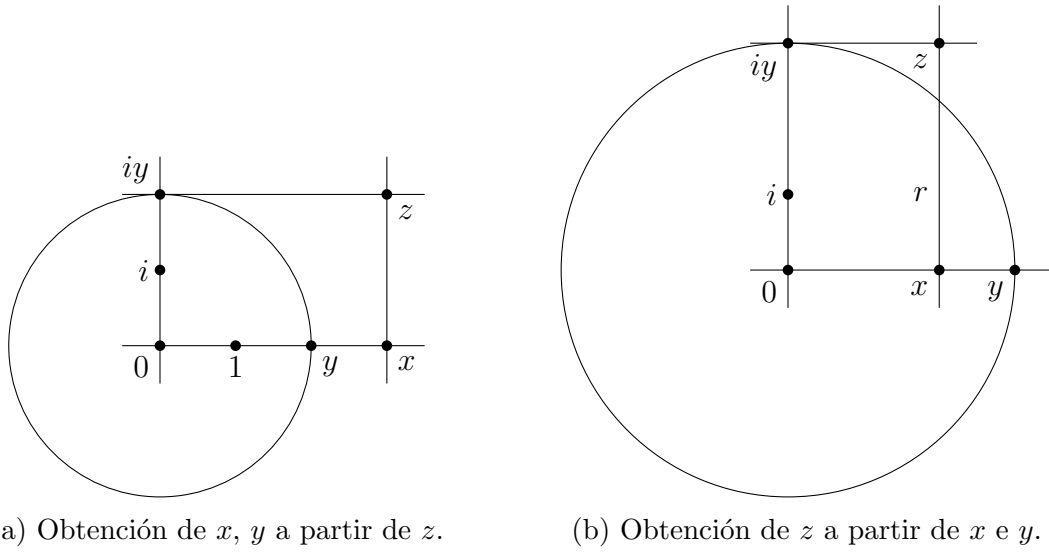
Figura 1.9: Relación geométrica entre z \in \mathbb{C} y sus componentes x e y .
